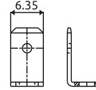
TERMINAL DETAYI ÖLÇEK 2/1
